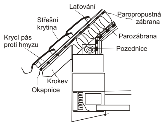
Napojení střechy
